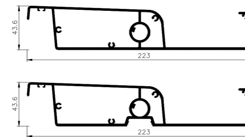
Lamela dachowa o wymiarach 44×223 mm
